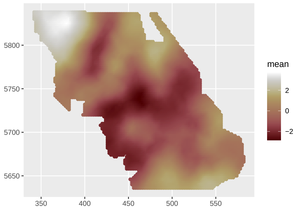
Posterior mean
