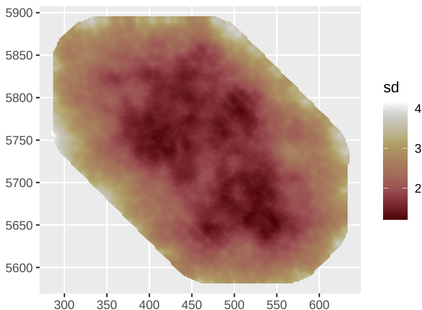
Posterior sd
