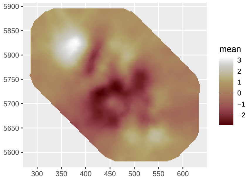
Posterior mean
